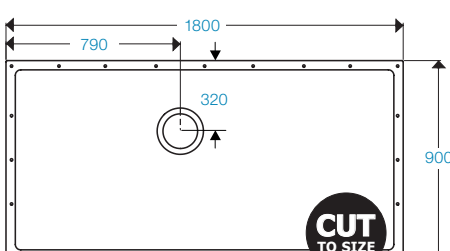
SHOWERDEC® 1800x900
