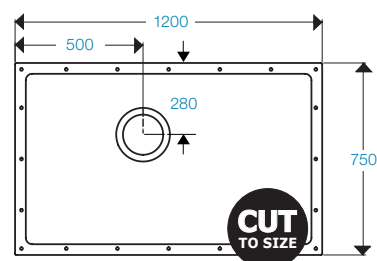
SHOWERDEC® 1200x750
