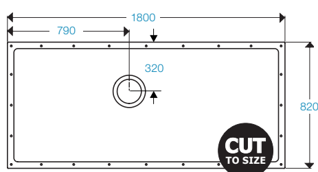
SHOWERDEC® 1800x820
