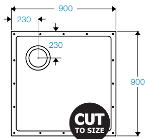
SHOWERDEC® 900x900
