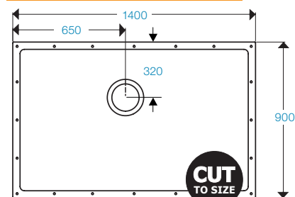
SHOWERDEC® 1400x900
