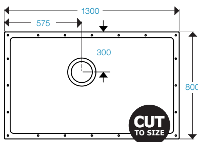
SHOWERDEC® 1300x800
