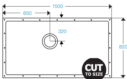
SHOWERDEC® 1500x820
